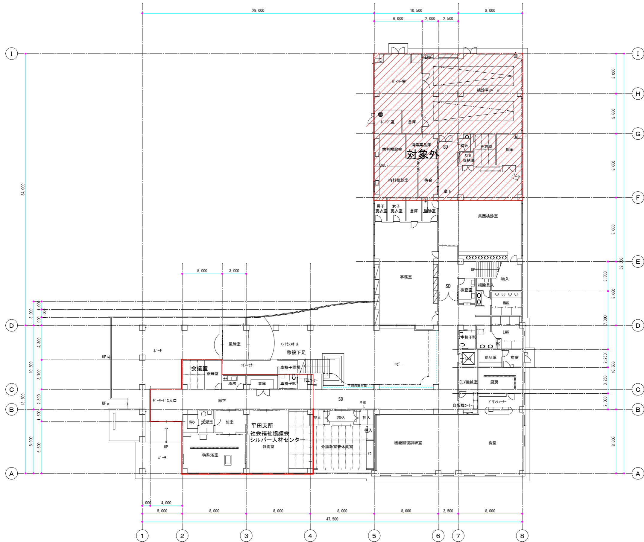
1階平面図
