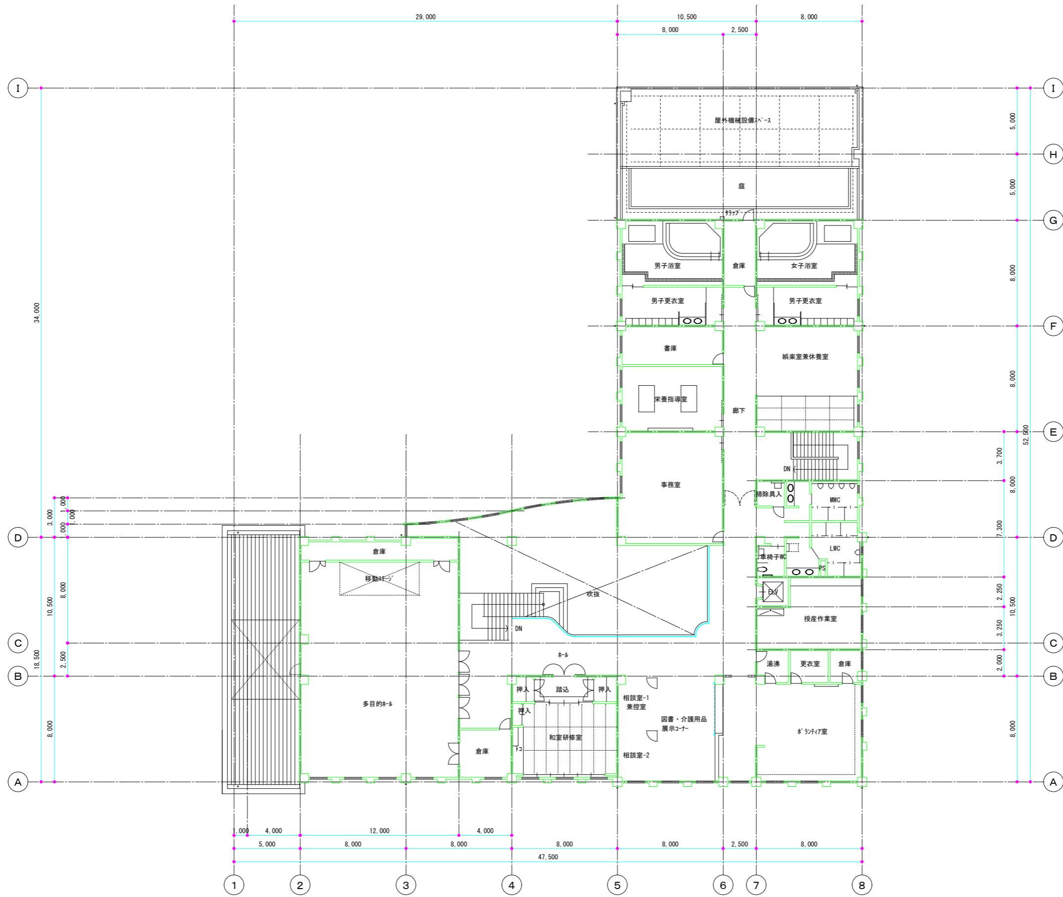
2階平面図
