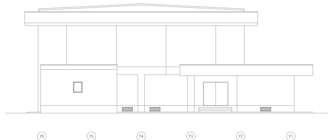
西立面图 1/200
