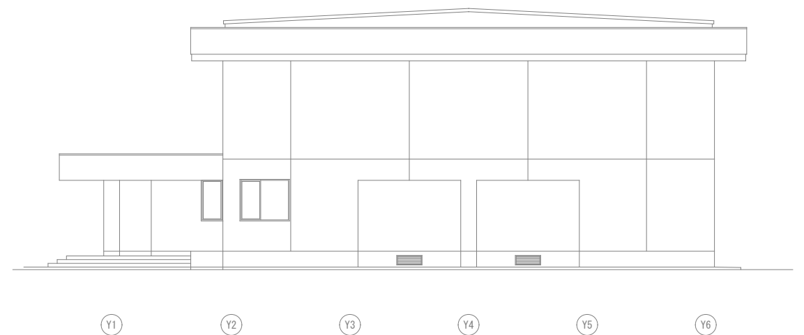
東立面図 1/200
