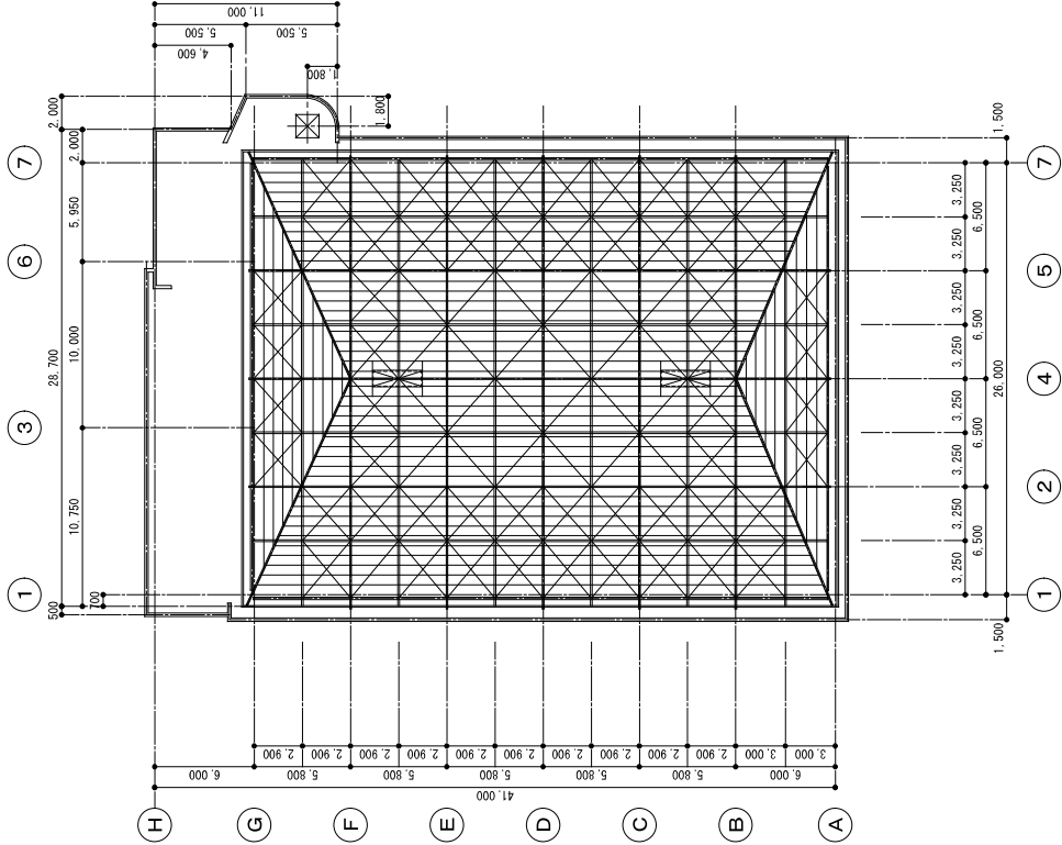
小屋伏図 S=1:250
