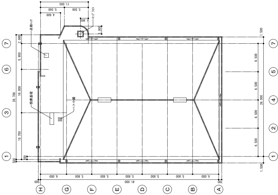
R階平面図 S=1:250
