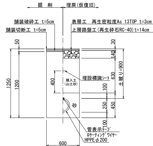
土工1-1 市道(車道) HPPE \phi 200 (土被り0.9m)
