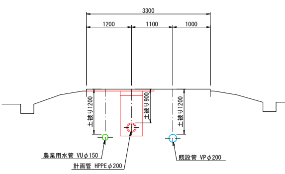
B - B 断面図 S=1:50
