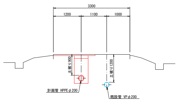
A - A 断面図 S=1:50
