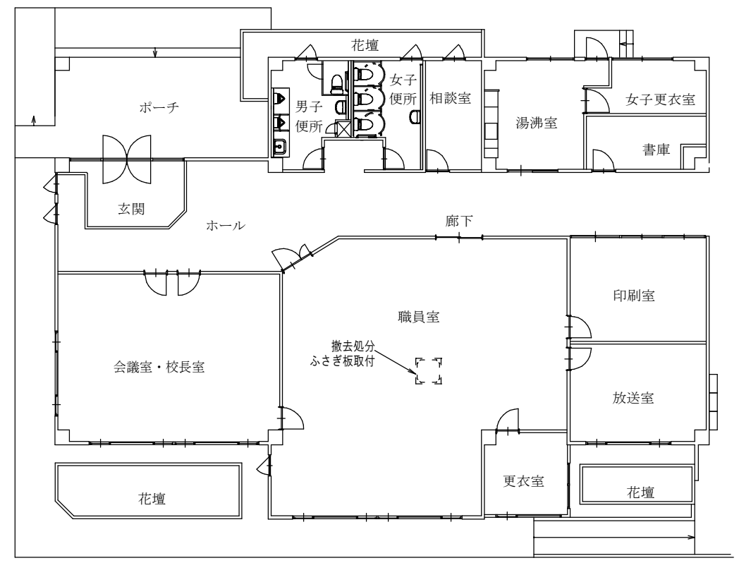
既設 撤去図面
