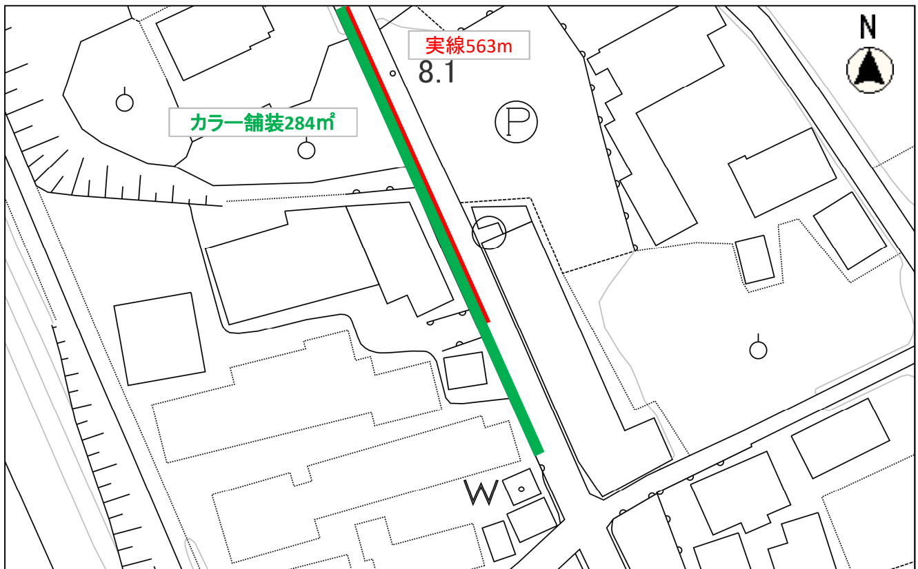
平面図(南端部)
