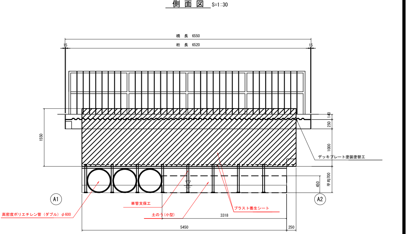
断面図 S=1:
