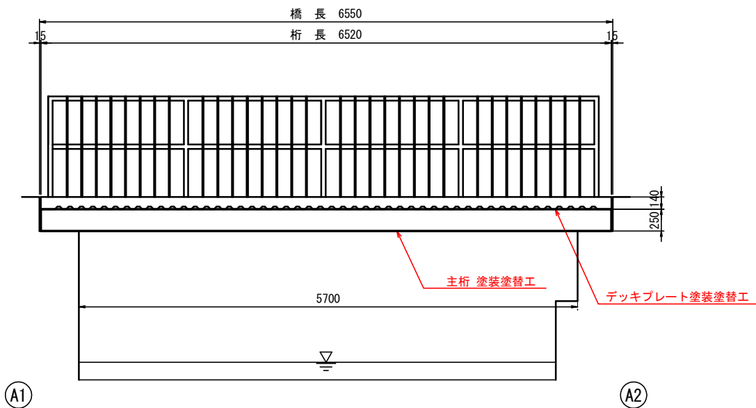
側面図 S=1:30
