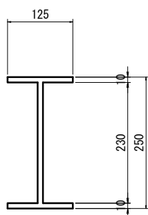
主桁 S=1:5
