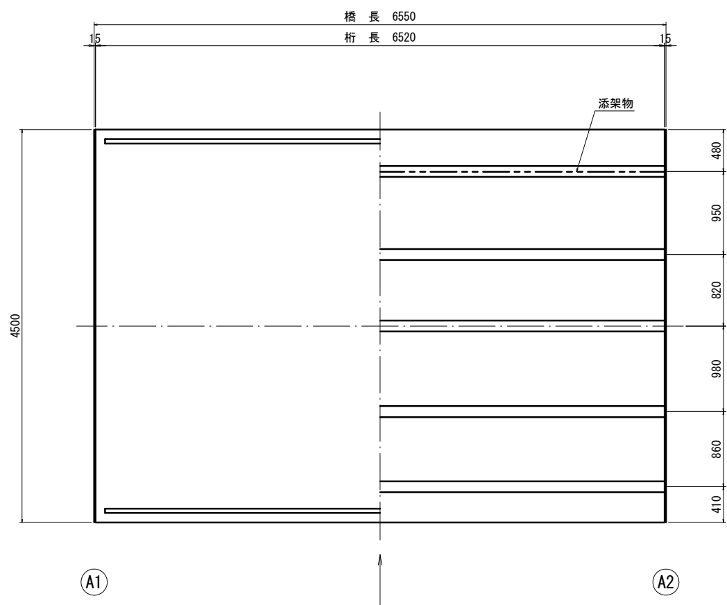
平面図
