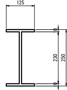
主桁 S=1:5
