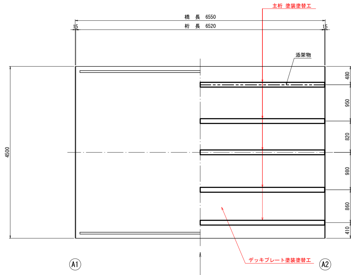
平面図 S=1:30
