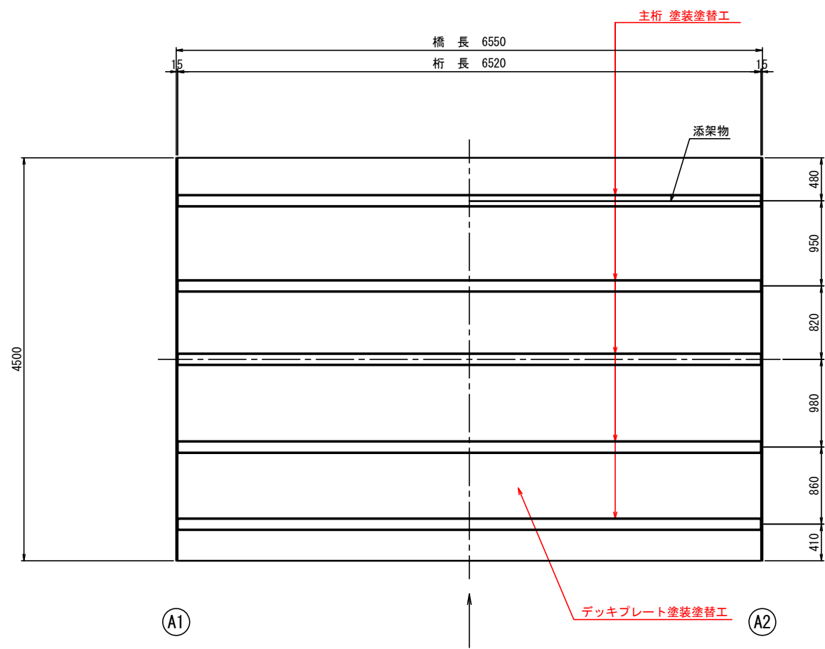
平面図 S=1:30
