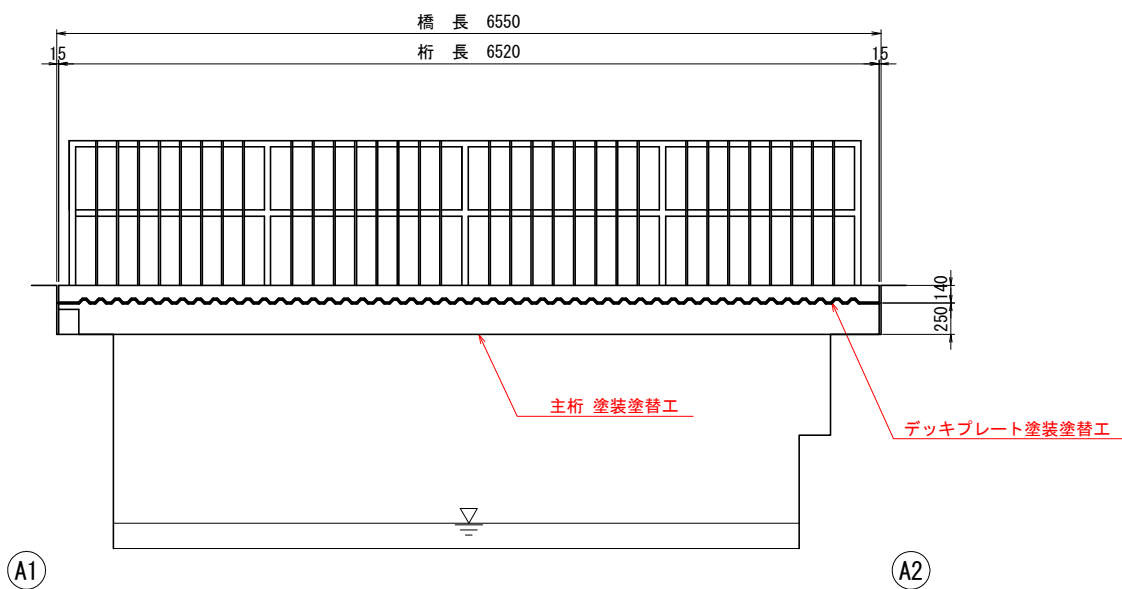
側面図 S=1:30
