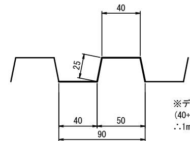
デッキプレート S=1:2
